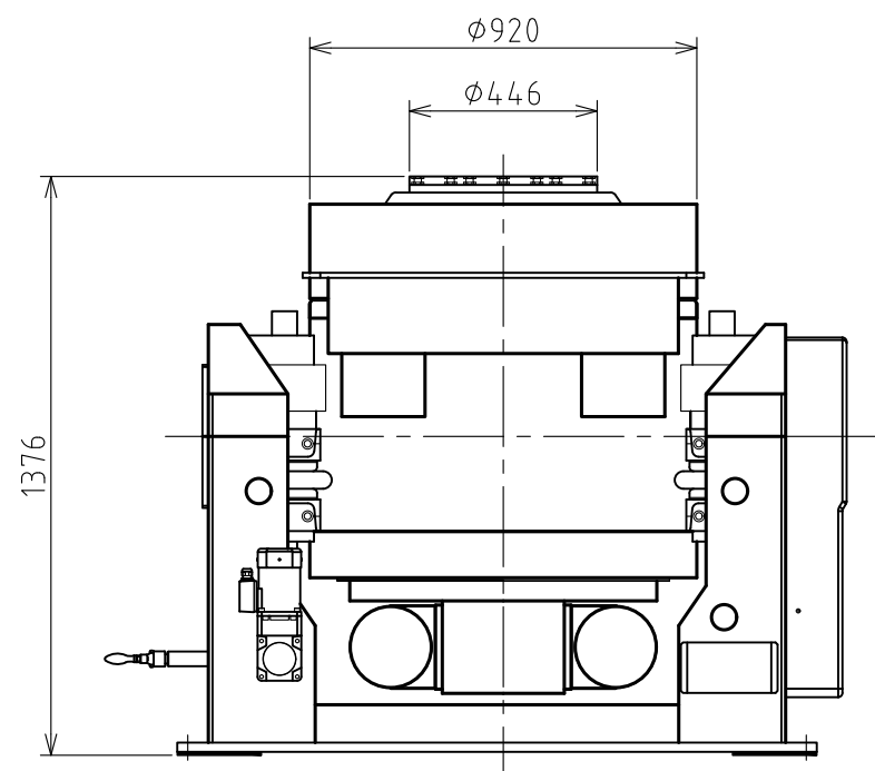
垂直加振時
