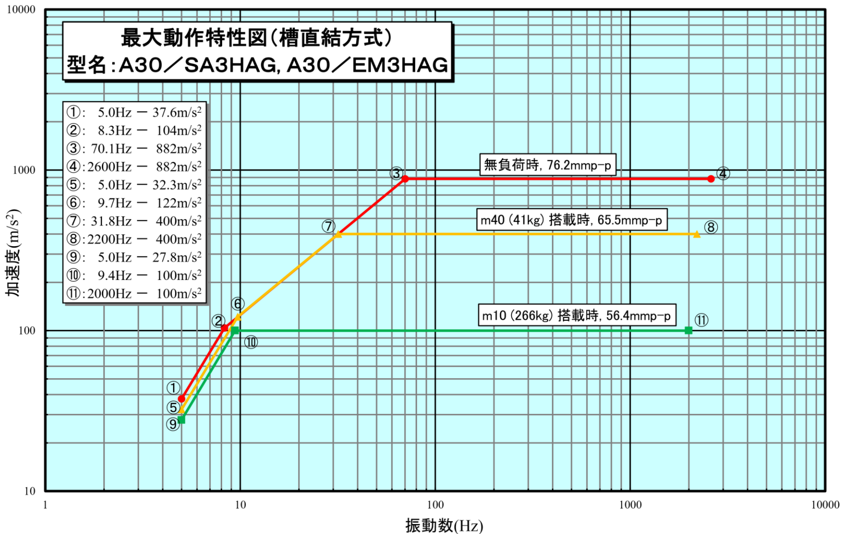
最大動作特性図 (槽直結方式) A30/SA3HAG
